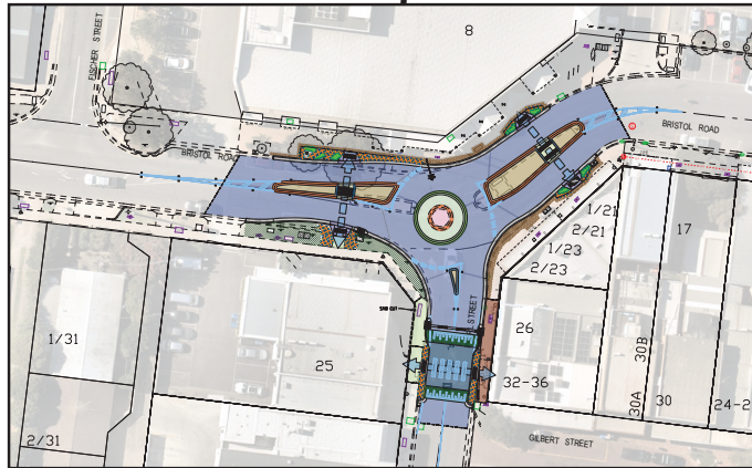
Mini roundabout plan - Bristol Rd and Pearl St.
